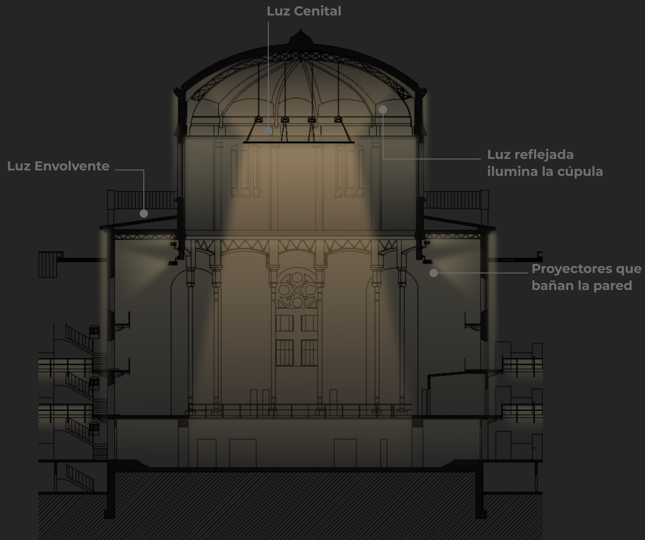
Sección
